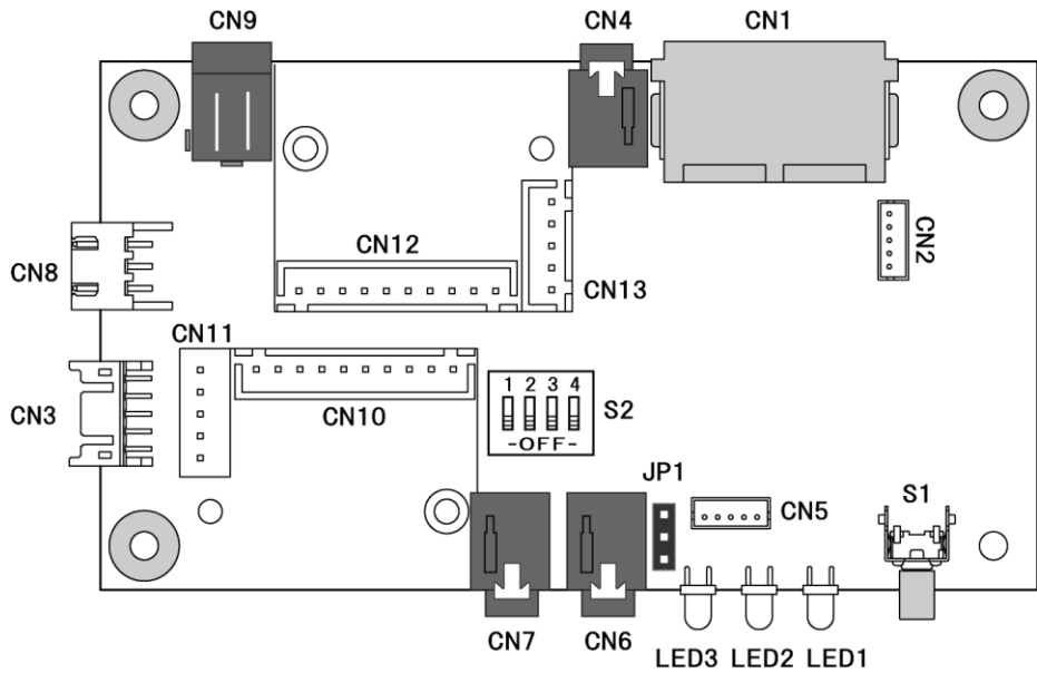
図5-1 コネクタ配置図
