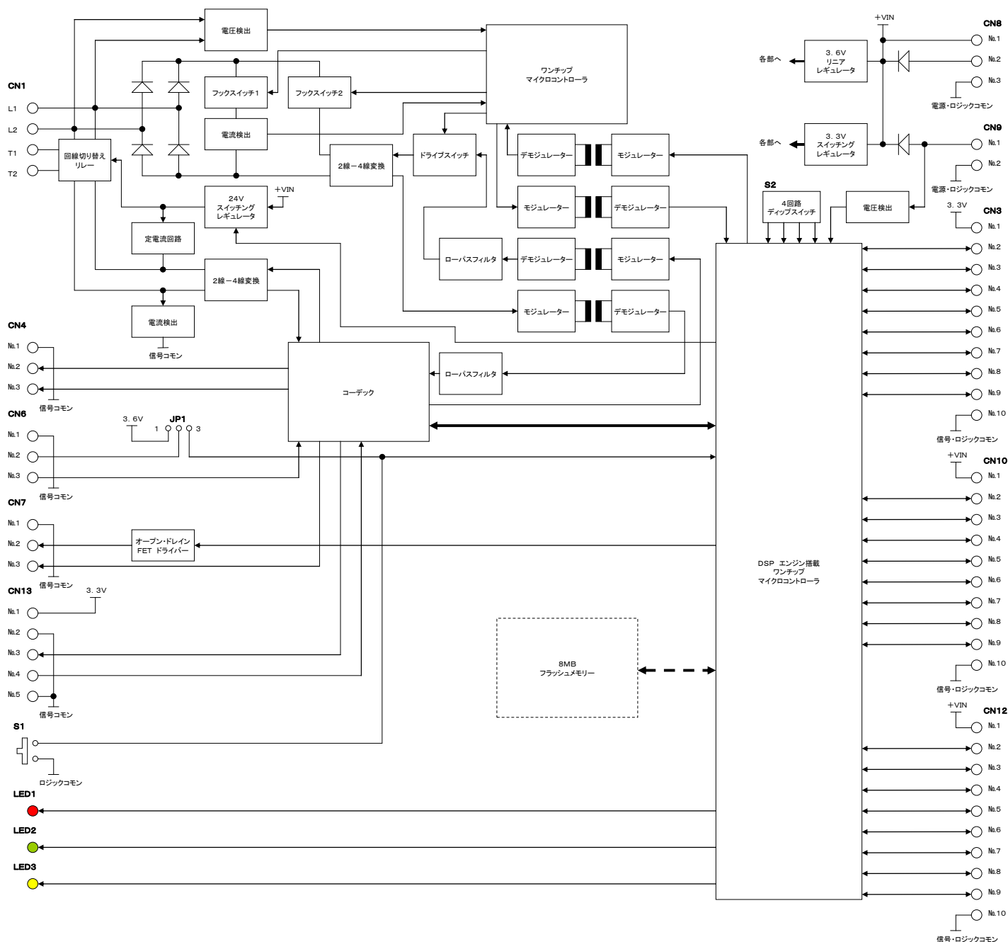
図4-3 ブロック図
